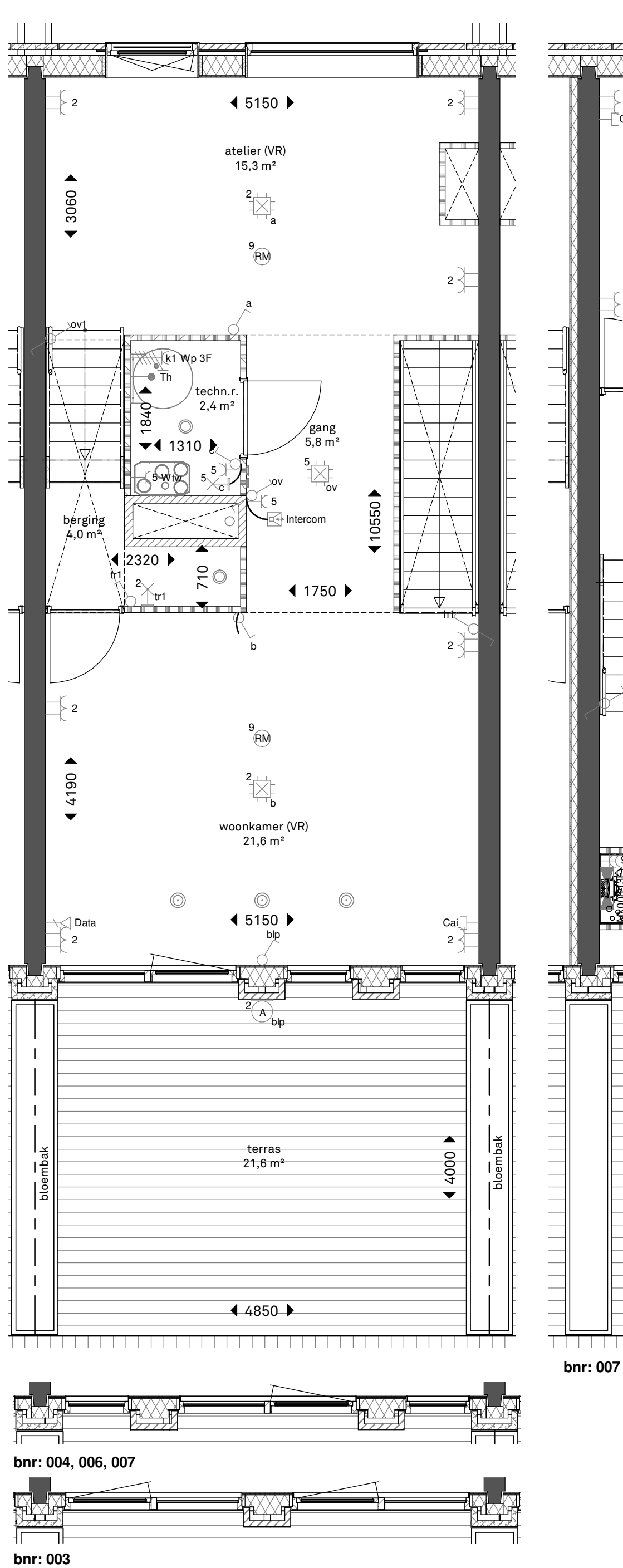
Woningtype A1 schaal 1 : 50
