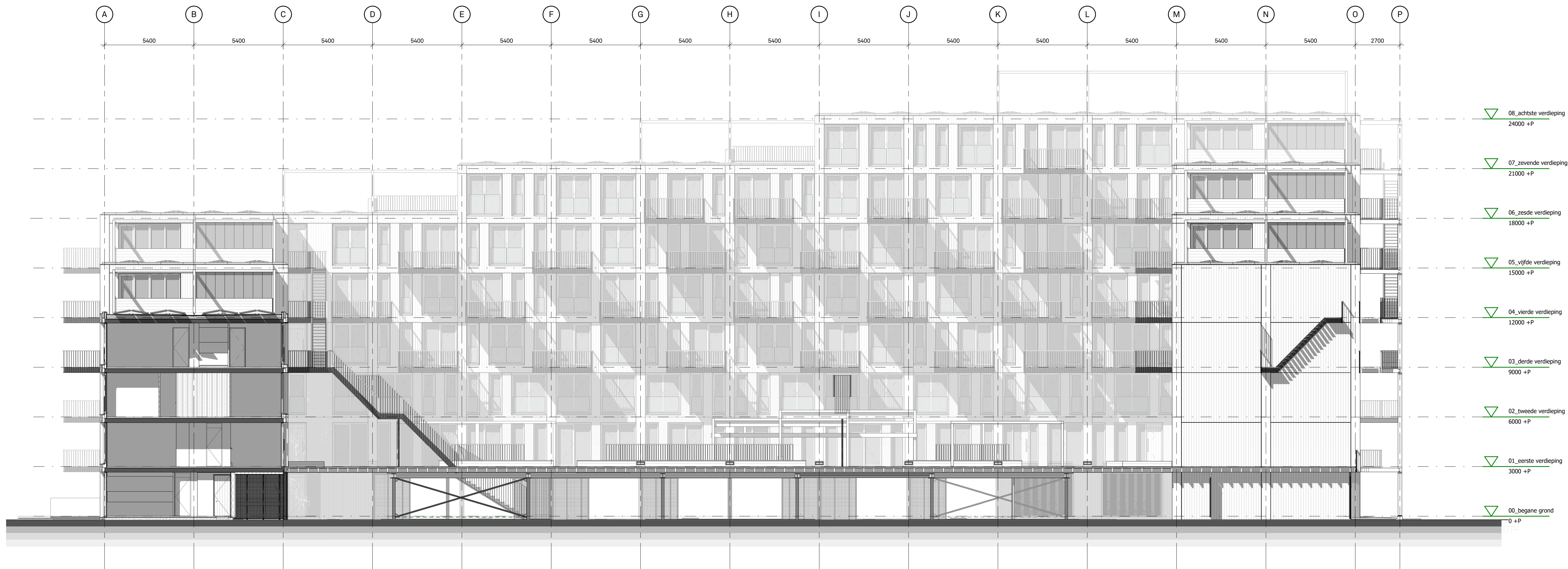
zuidgevel corridor binnenzijde
