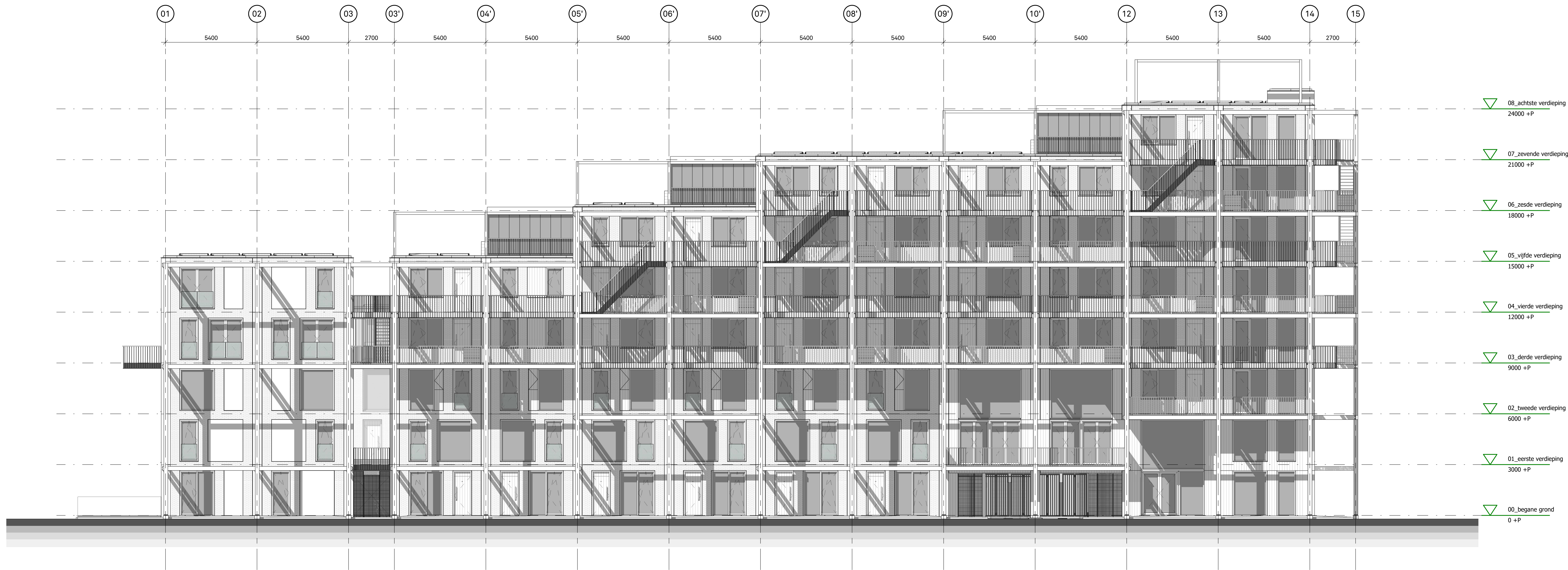
oostgevel schaal 1 : 100
