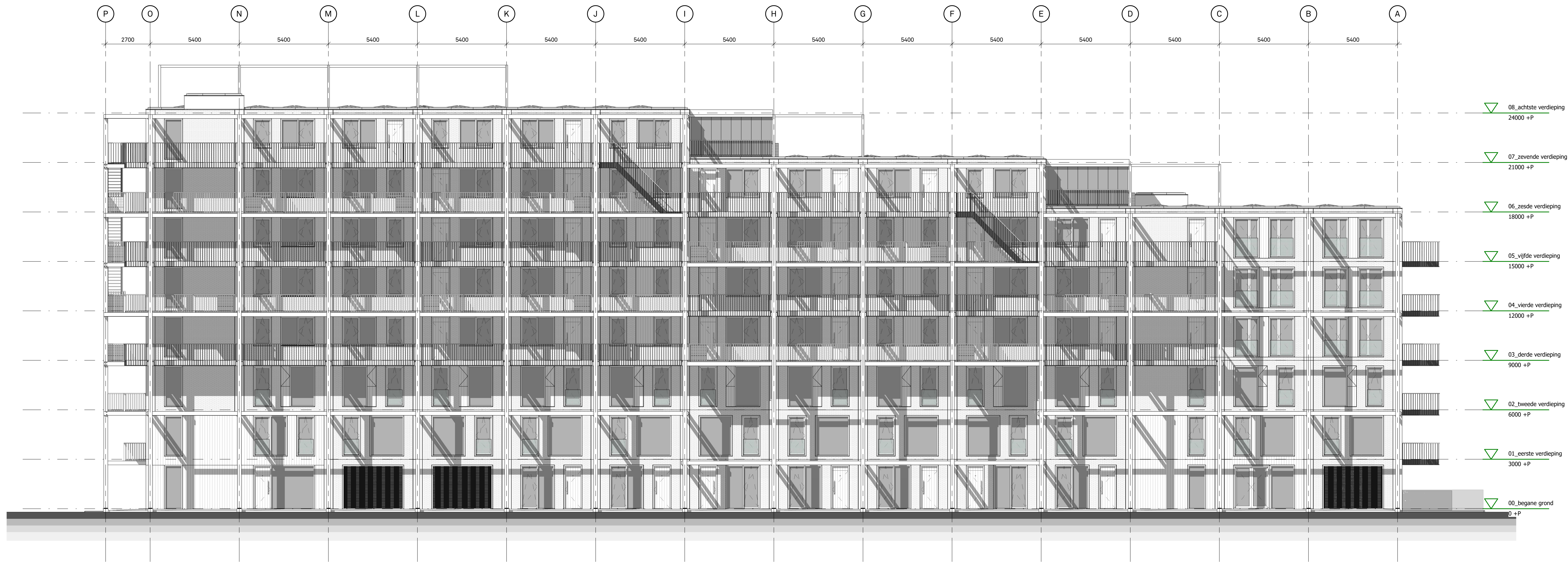
noordgevel schaal 1 : 100
